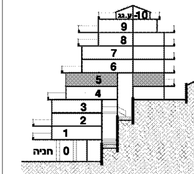
חצר סכמתי
