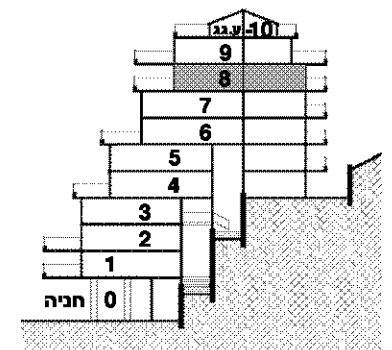
חתך סכמתי
