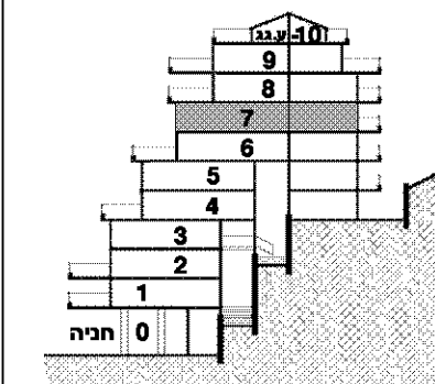
חתך סכמתי
