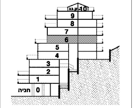
חתך סכמתי ייתכנו שינויים והתאמות בשל דרישות הרשויות, המתכננים והיועצים. יש לקרוא את התכנית יחד עם הערות ומקרא סימונים המופיעים בדף הערות ובצמוד למפרט מכר.
